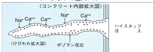
ハイスタッフの注入メカニズム
