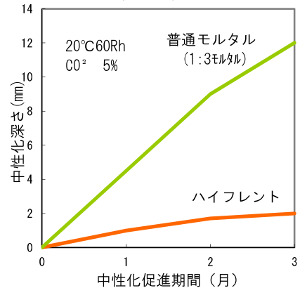
中性化試験
