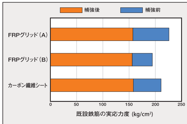
補強前後の既設鉄筋の実応力度の変化
