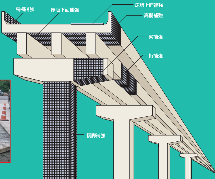
(ポリマーセメントモルタル吹付工)
