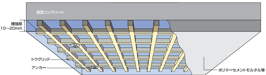
■施工概念図
