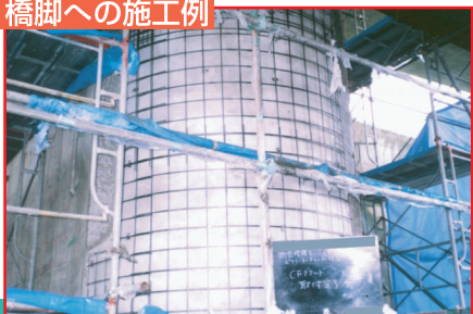
橋脚への施工例
