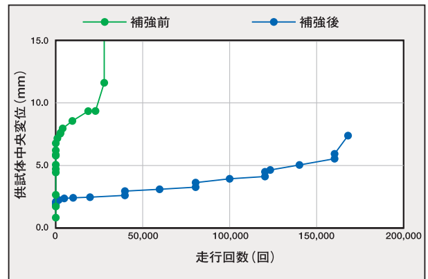
変位と走行回数との関係 (載荷時)
