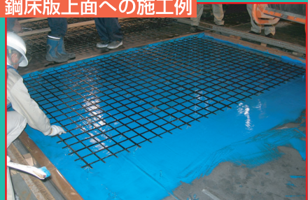
鋼床版上面への施工例
